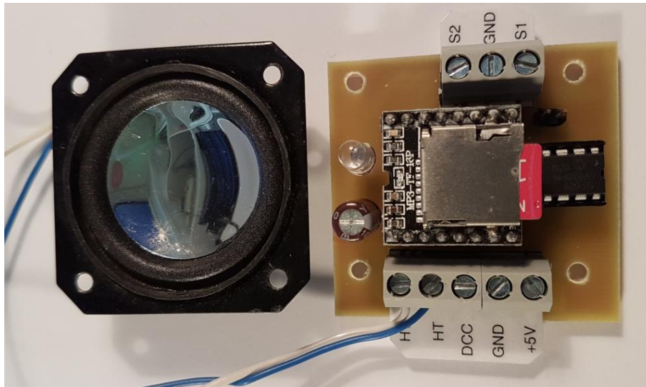
Komponentside
